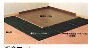
遮音マット
